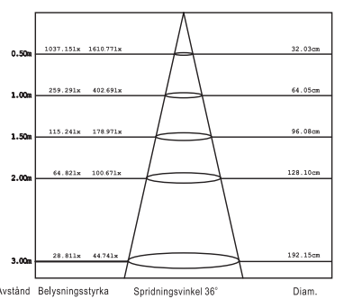
Avstånd Belysningsstyrka Spridningsvinkel 36° Diam.
